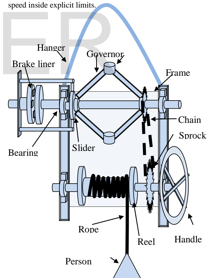
Fig. 2.General Layout
